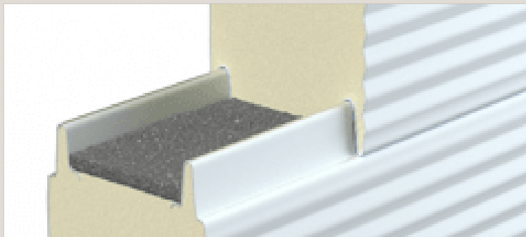
Aansluiting (zichtbare bevestiging, dikte 60 - 100mm)
