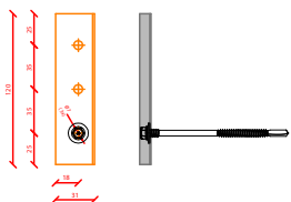
Drukverdeelplaat PREMIUM ALPHA-AR CORTEN Afmeting: 120* 31* 9* 1,5 Artikelnr.: 1008906
