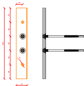
Drukverdeelplaat PREMIUM ALPHA-AR CORTEN Afmeting: 200* 31* 9* 1,5 Artikelnr.: 1009059
