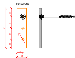
Drukverdeelplaat PREMIUM ALPHA-AR CORTEN Afmeting: 120* 31* 9* 1,5 Artikelnr.: 1008906
