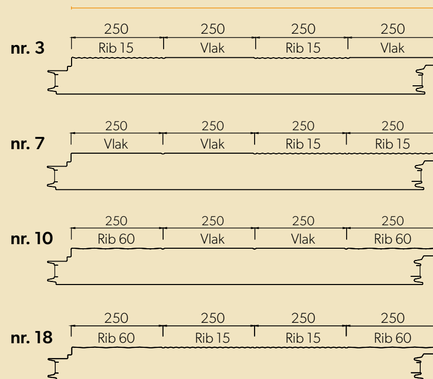
PROFIELVARIANTEN (voorbeelden)
