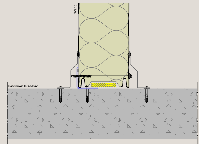
Principedetail scheidingswand
