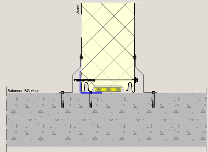
Principedetail scheidingswand
