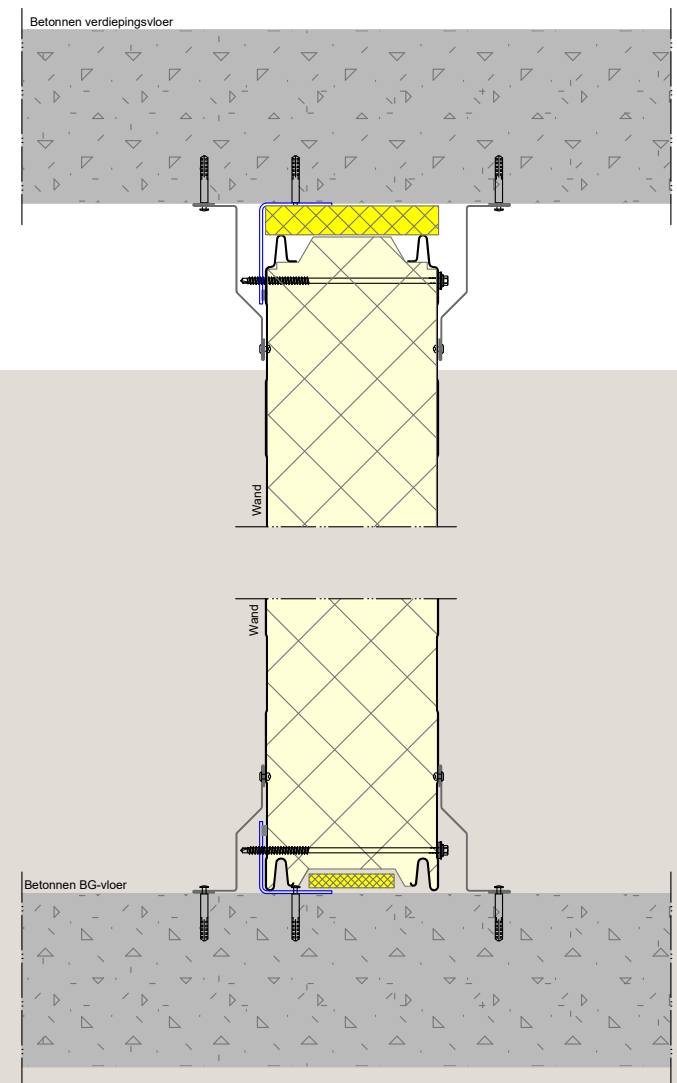
Principedetail scheidingswand
