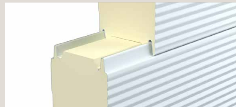
Aansluiting (zichtbare bevestiging, dikte 120 - 200mm)
