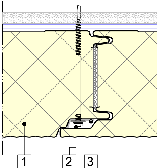
Horizontale doorsnede
