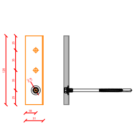
Drukverdeelplaat Alpha-PR FX Afmeting: 120* 31* 9* 1,5 Artikelnr.: 1008906
