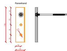
Drukverdeelplaat Alpha-PR FX Afmeting: 120* 31* 9* 1,5 Artikelnr.: 1008906
