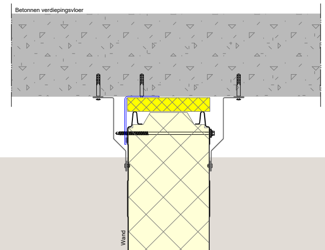
Principedetail scheidingswand
