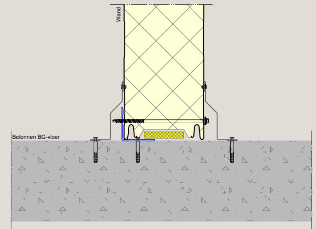
Principedetail scheidingswand
